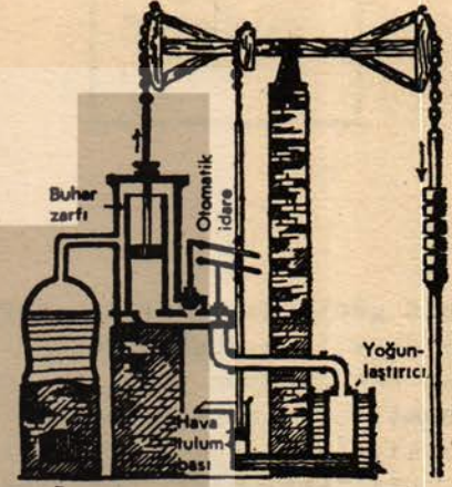
Watt'ın John Wilkinson için Birminham'da kurduğu ilk buhar makinesi.
